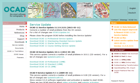
Fig. 3: Uppgradering
