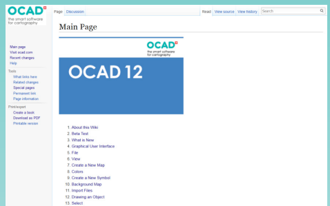
Fig. 2: Hjälp
