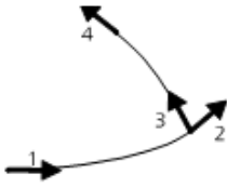
Fig. 5: Nodo d'angolo per creare una cuspidi lungo una Curva di Bézier
