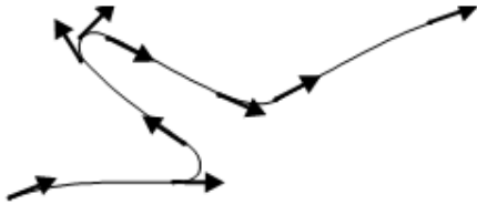
Fig. 2: Punti di curvatura (flessi) di una curva di Bézier
